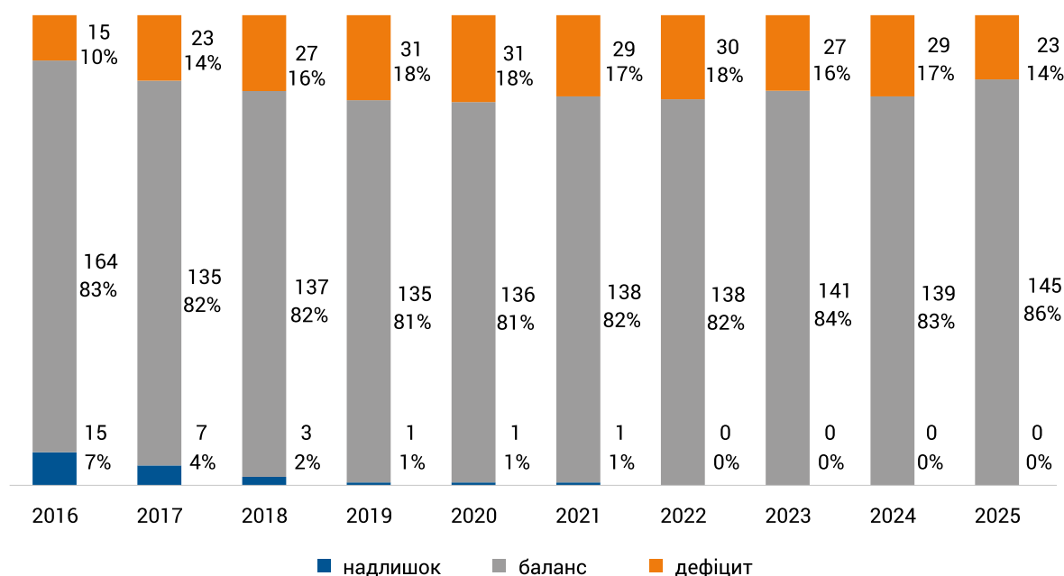
Діаграма 2. Кількість та частка дефіцитних, збалансованих та надлишкових професій у Барометрі професій у прогнозах на 2016–2025 рр.
